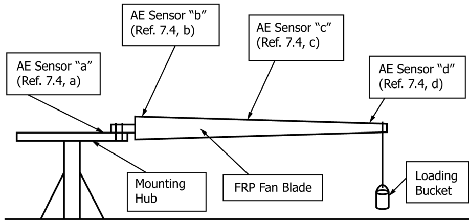
FIG. 1 Apparatus
