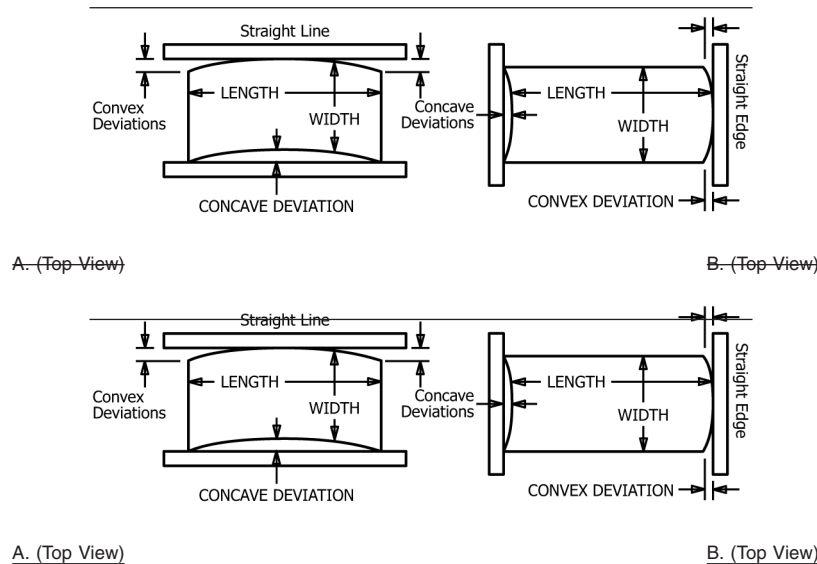
FIG. 1 Edge Trueness
