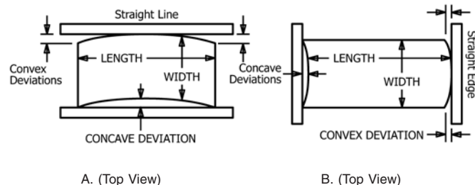
FIG. 1 Edge Trueness
