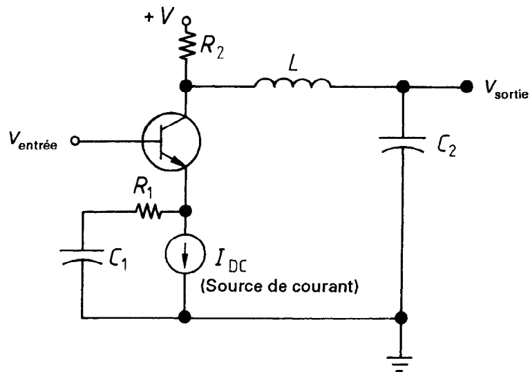
Figure A.1 — Exemple d'amplificateur-différentiel
