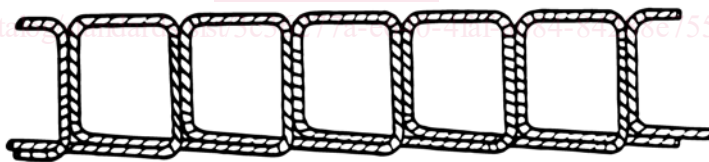
FIG. 7 Stitch Type 202
