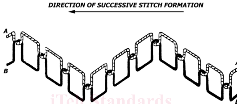
FIG. 24 Stitch Type 314
