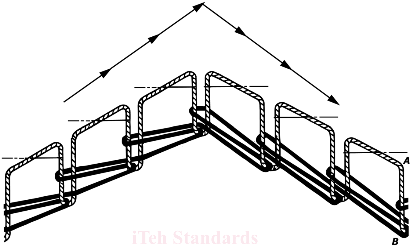
FIG. 35 Stitch Type 409
