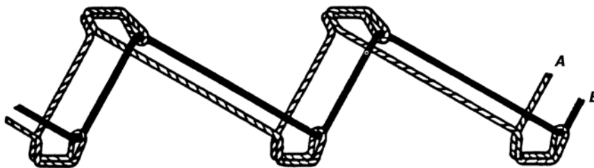
FIG. 23 Stitch Type 313
