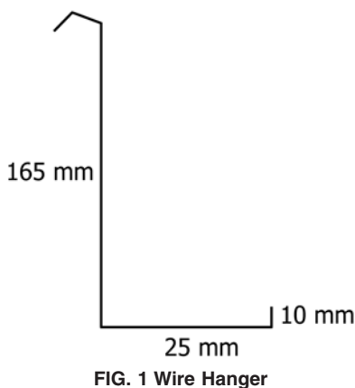
FIG. 1 Wire Hanger
