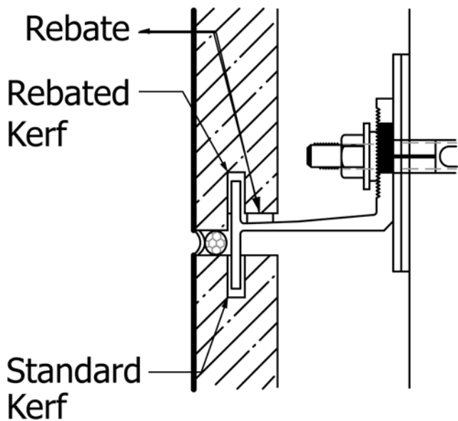
FIG. 3 Rebated Kerf
