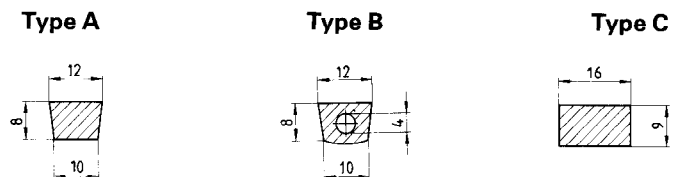
Figure 1 — Coupes transversales des joints
