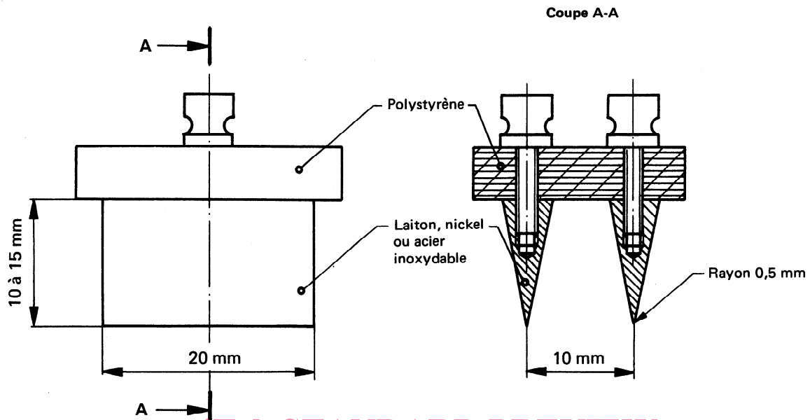
Figure 2 — Électrodes potentiométriques (standards.iteh.ai)
