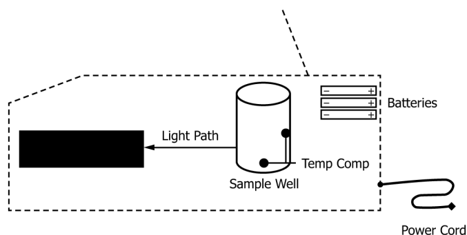
FIG. 1 Luminometer
