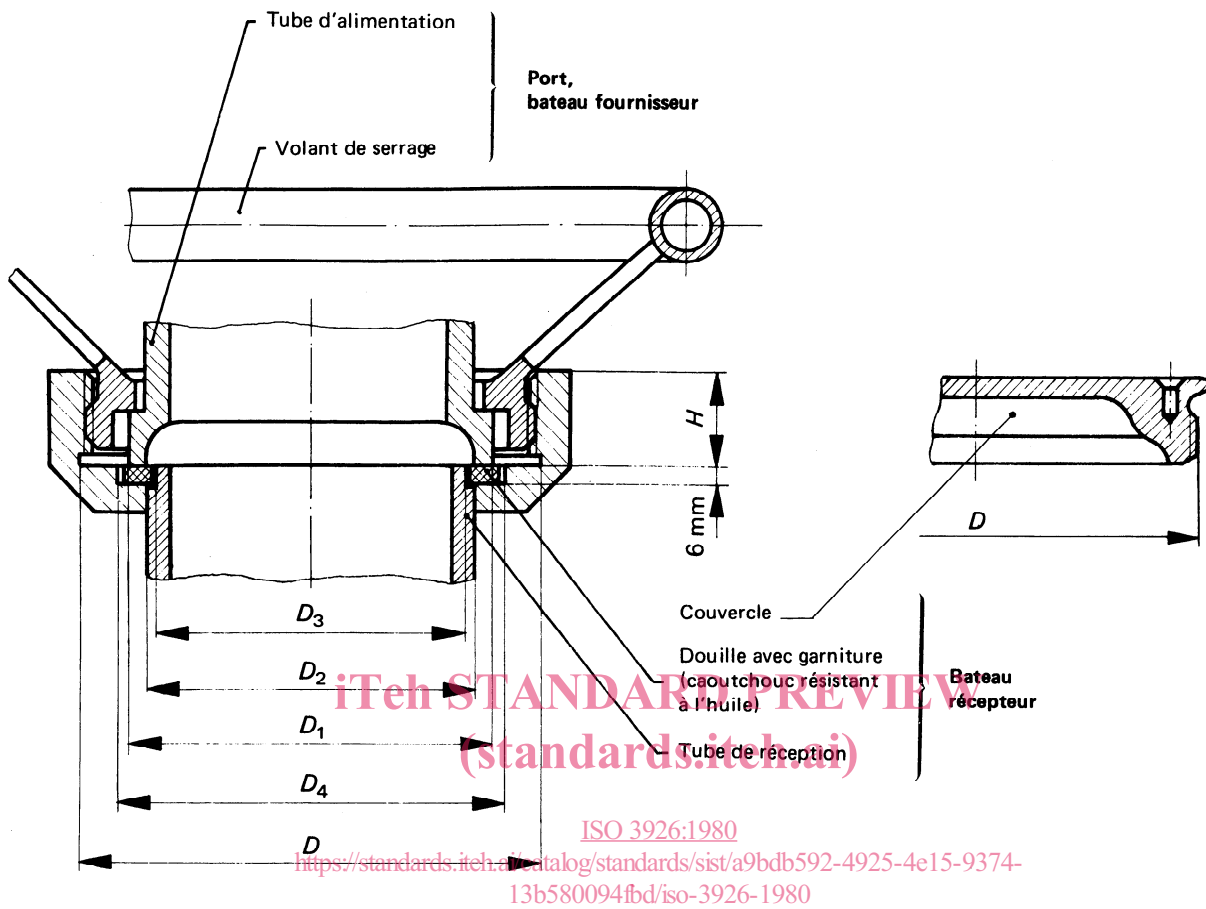
Figure 1 — Dispositif de réception d'huile et de combustible pour les dimensions nominales 50 et 80
