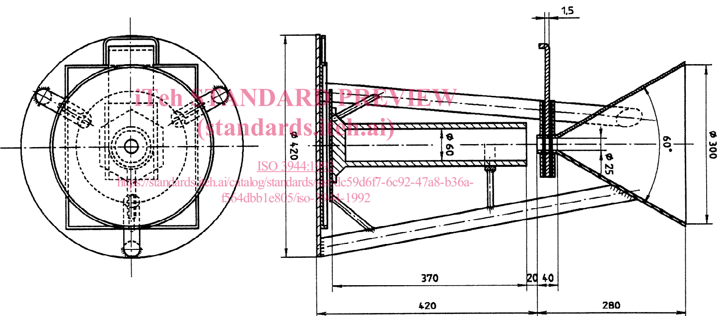
Figure 1 — Appareil pour la détermination de la masse volumique sans tassement
