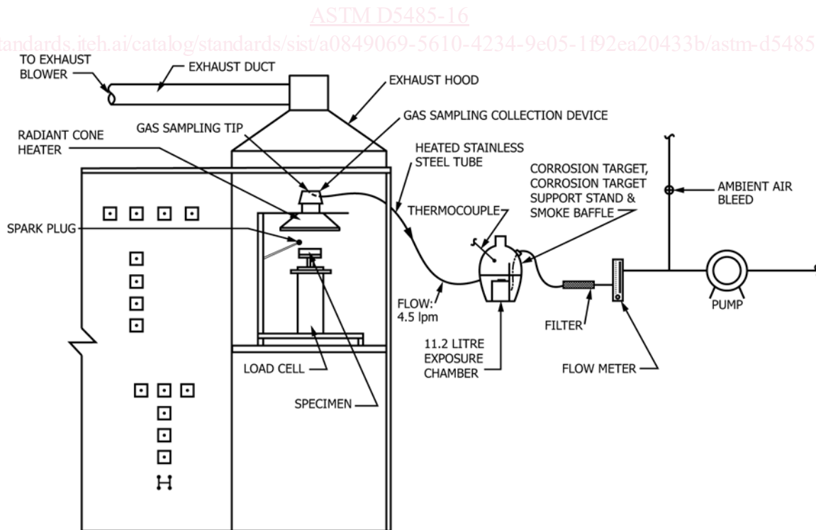
FIG. 1 Cone Corrosimeter
