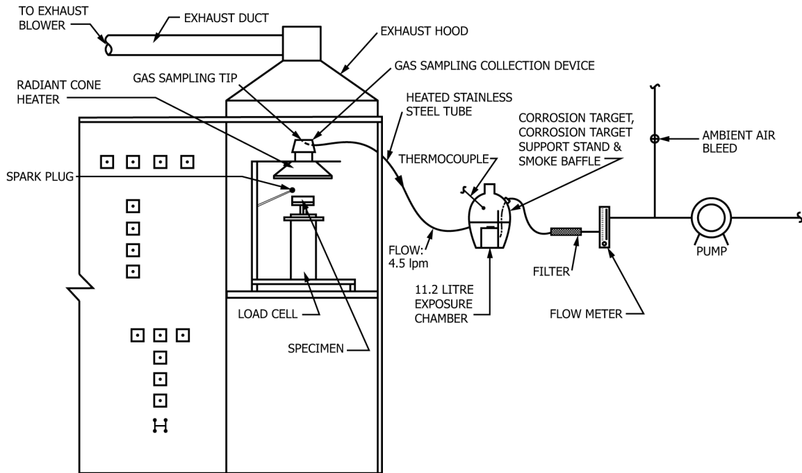
FIG. 1 Cone Corrosimeter
