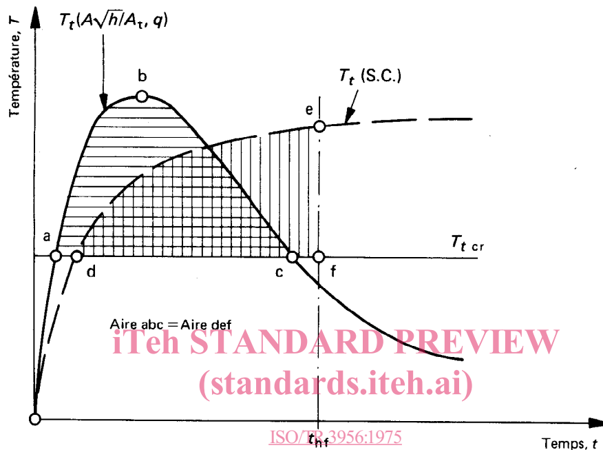
FIGURE 3 – Détermination de la durée de feu empirique selon la méthode des aires égales
