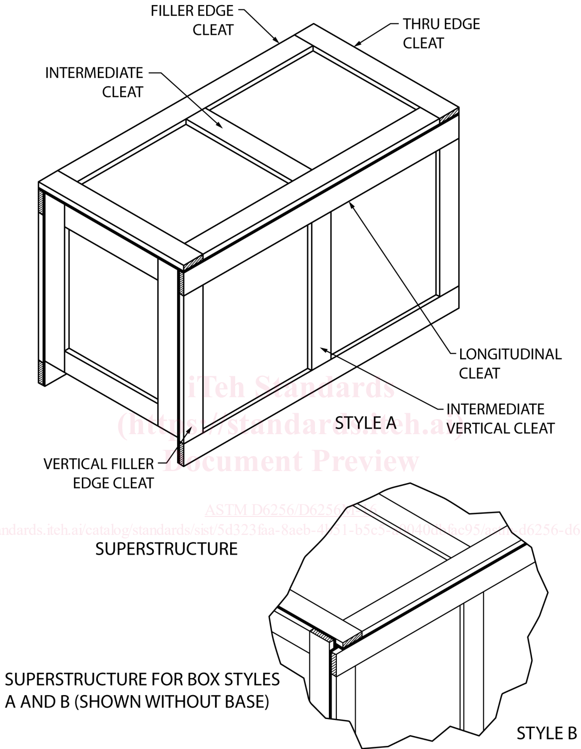
FIG. 2 Box Styles
