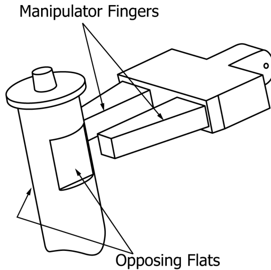
FIG. 2 Machined Flats
