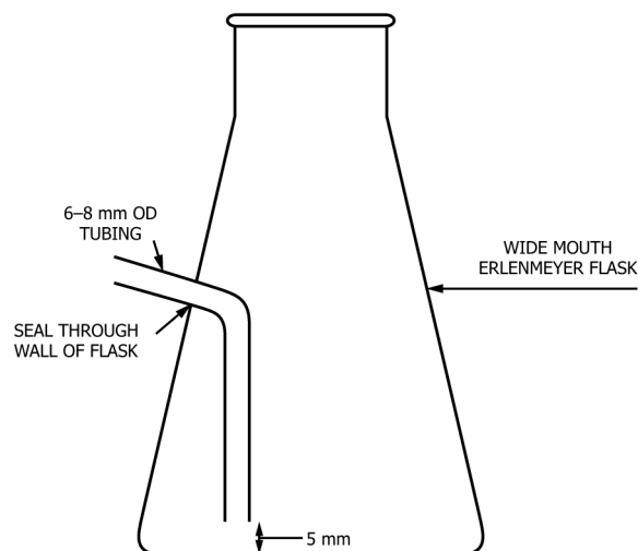
FIG. 1 Titration Flask
