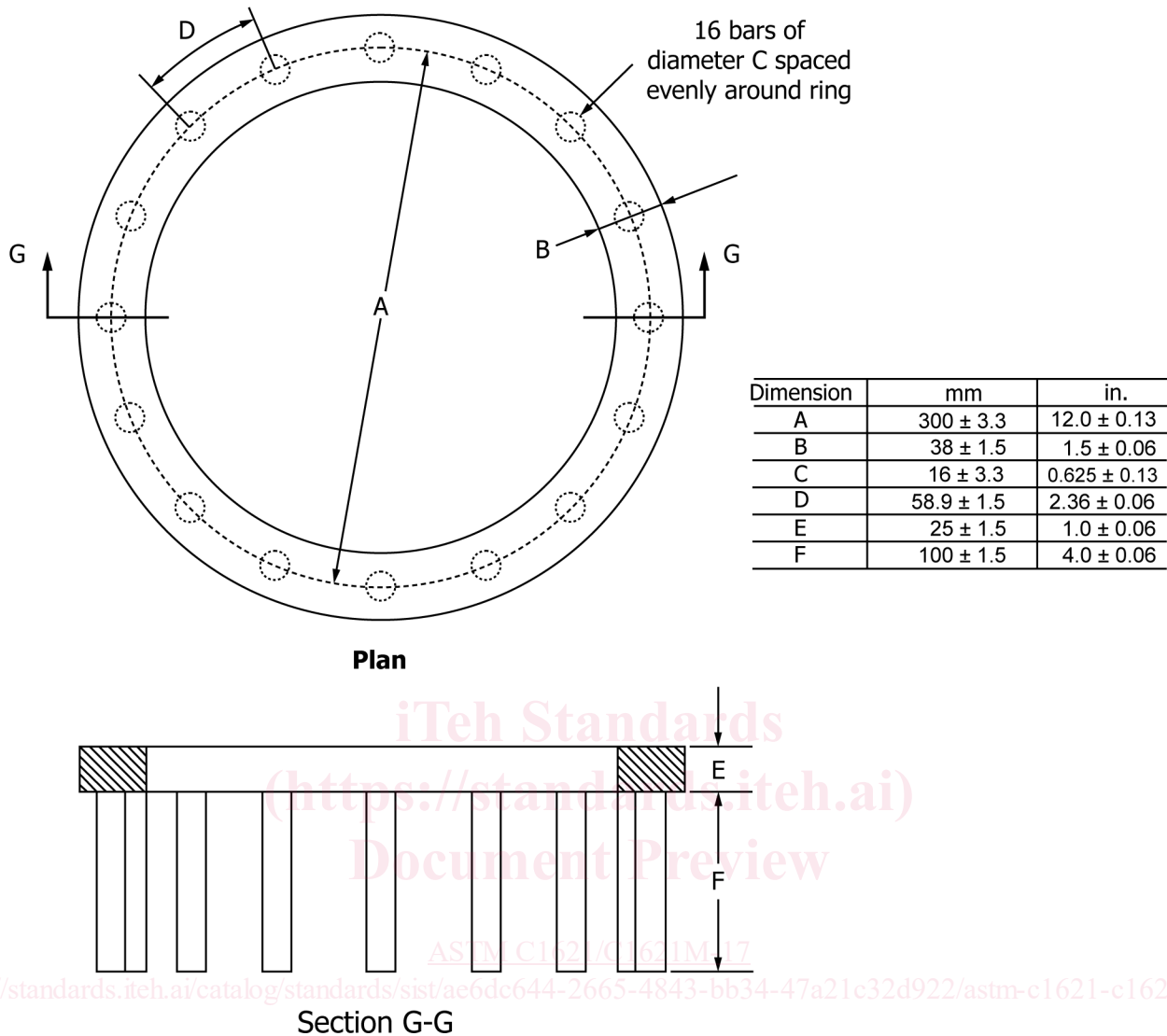
FIG. 1 J-Ring Apparatus
