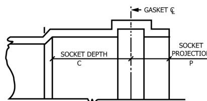
FIG. 1 Gasket-Joint Dimensions
