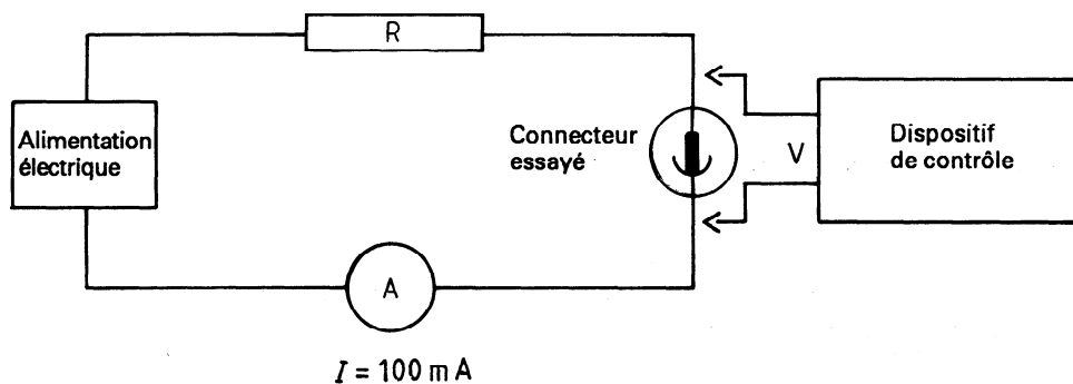
Figure 2 — Contrôle de la résistance de contact
