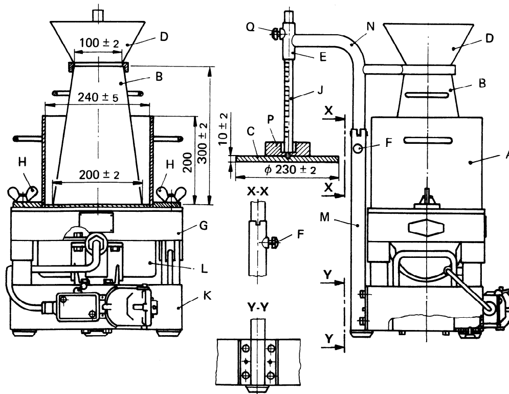
Figure — Consistomètre (appareillage Vébé)
