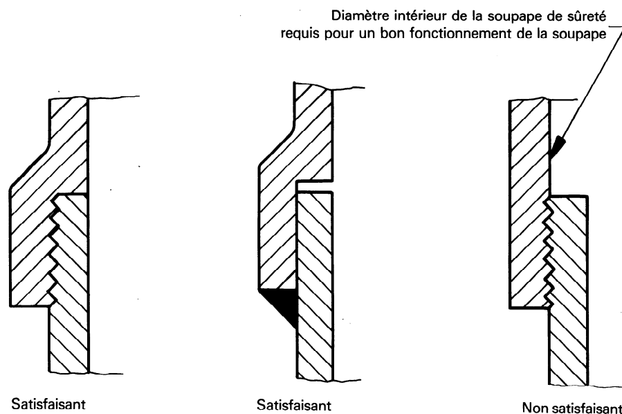
Figure 1 — Configuration des raccords d'extrémité
