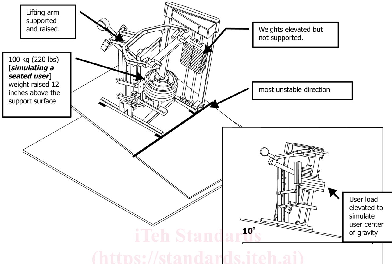
FIG. 1 Tilt Test
