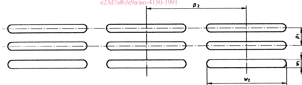
Figure B.1 — Tamis à trous longs arrondis — Disposition en lignes
