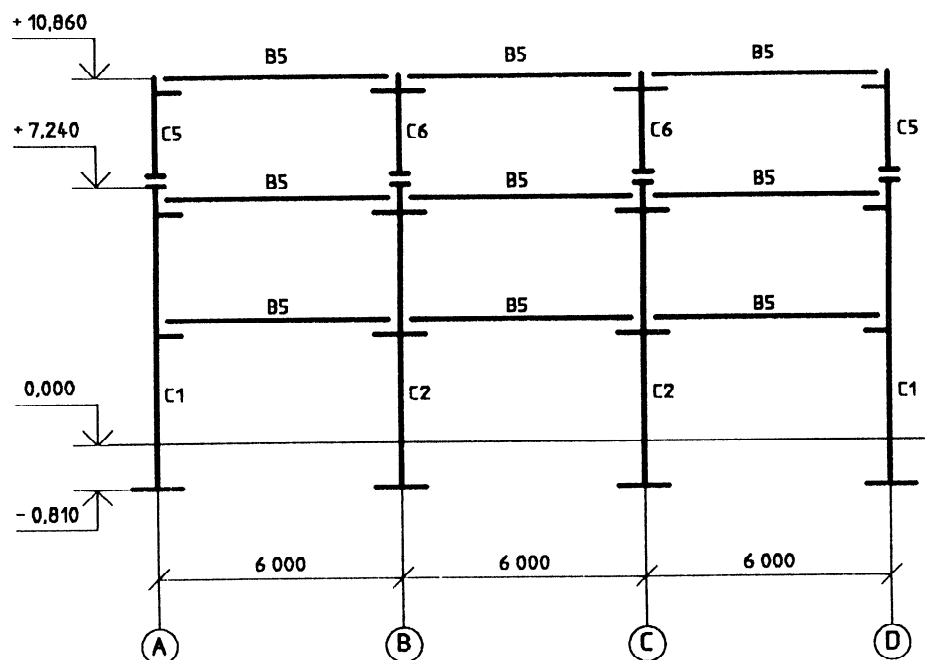
Figure 4 – Exemple de section type (échelle 1 : 200) itih STANDARD PREVIEW (standards.iteh.ai)
