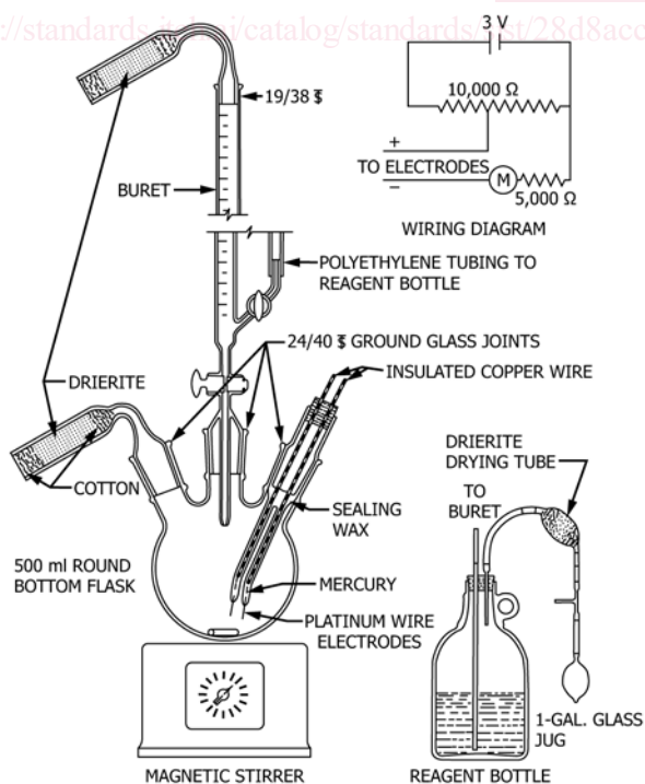
FIG. 1 Titration Assembly
