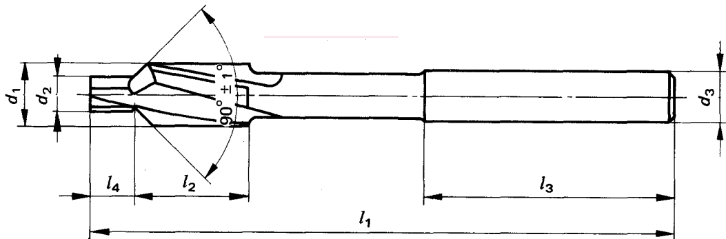
L'illustration représente un outil à chanfreiner de diamètre d_1 supérieur à 5 mm.
