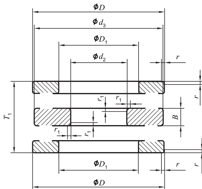
Figure 2 — Butée rondelles plates à double effet
