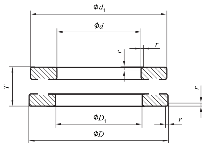
Figure 1 — Butée rondelles plates à simple effet
