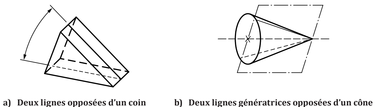
Figure 2 — Exemples d'entités dimensionnelles angulaires
