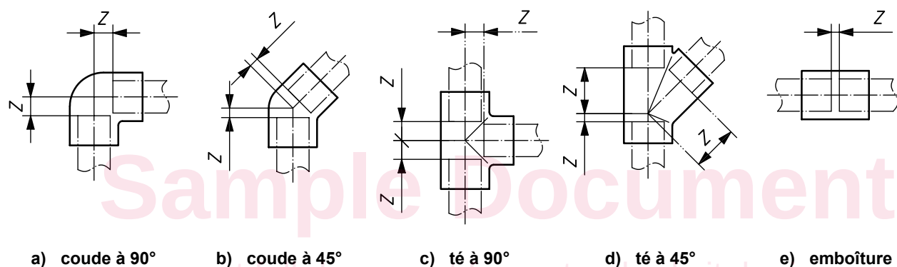
Figure 1 — Types de raccords: Coudes, tés et double manchon types
