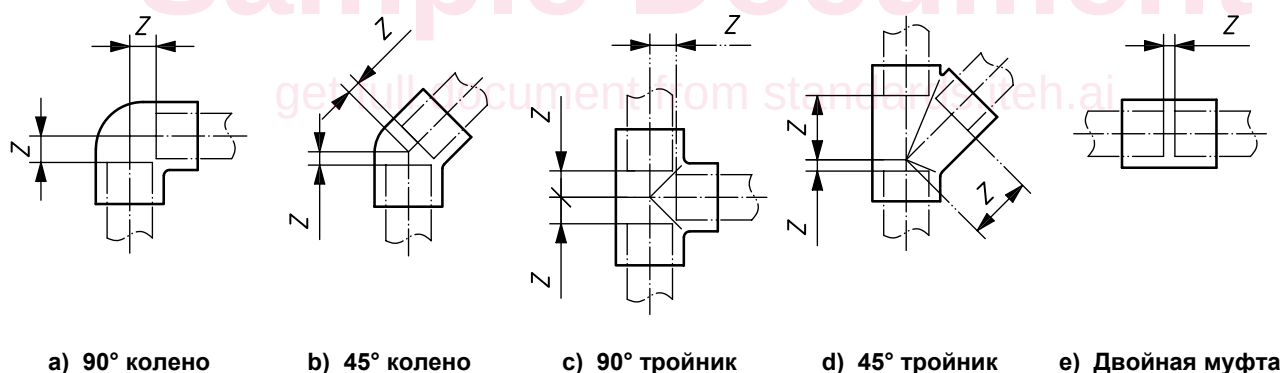
Рисунок 1 — Типы фитингов: Типичные колена, тройники и двойная муфта
