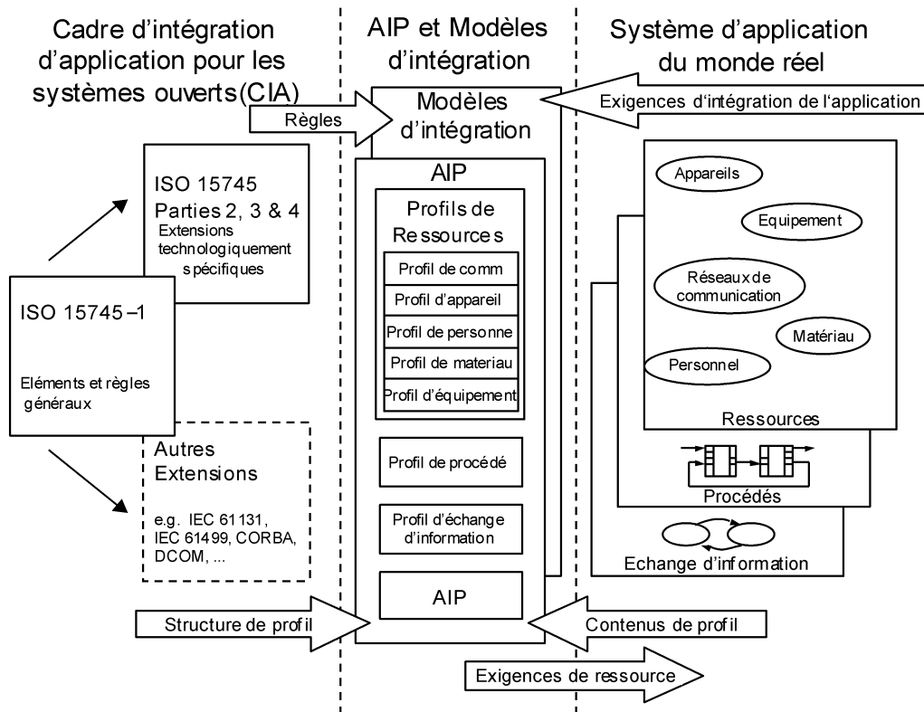
Figure 1 — Contexte de l'ISO 15745
