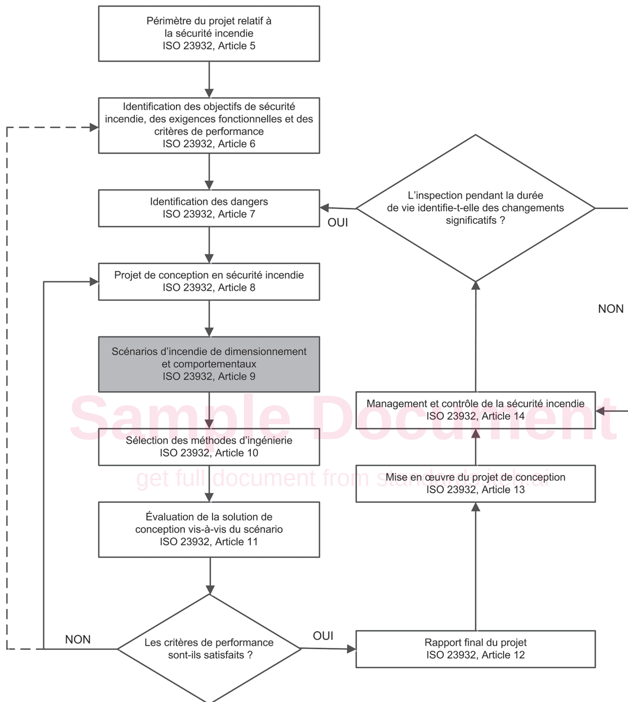
Figure 1 — Diagramme illustrant le processus d'ingénierie de la sécurité incendie ainsi que la sélection de scénarios d'incendie de dimensionnement (Source: ISO 23932:2009)
