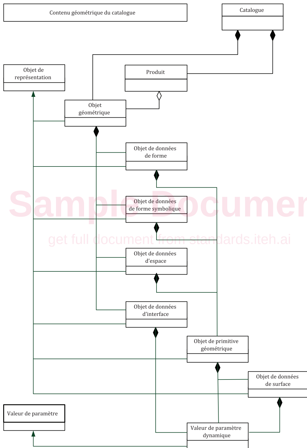
Figure 2 — Vue d'ensemble des éléments géométriques d'un catalogue et des types d'objets de données
