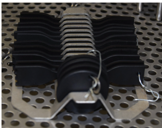
Figure 1 — Exemple de support d'éprouvettes avec plateaux et éprouvettes (éprouvettes haltère de type 2 et disques)
