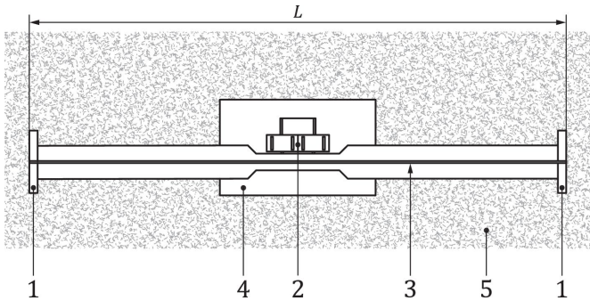
c) Jauge de déformation noyée
