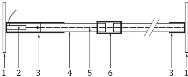
Figure 1 — Caractéristiques des jauges de déformation à corde vibrante
