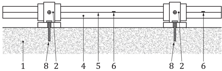
c) Jauge FBG de déformation boulonnée
