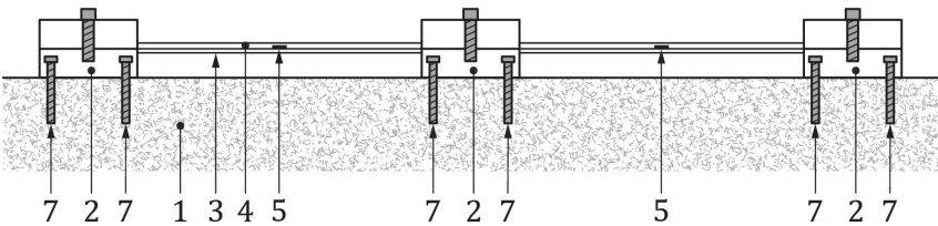
a) Réseau de FBG de déformation fixé par collier (installation sur la longueur entre repères)
