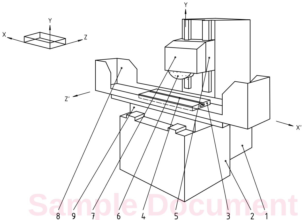
Figure 1 — Schéma d'une machine à rectifier les surfaces planes, à broche porte-meules à axe horizontal et table alternative
