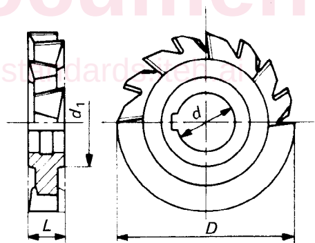
FIGURE 2 — Fraise à denture en double hélice alternée
