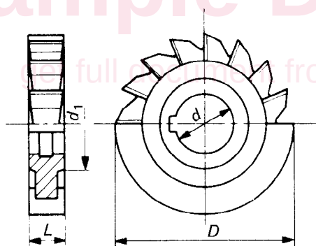
FIGURE 1 — Fraise à denture droite
