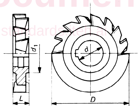
FIGURE 2 — Fraise à denture en double hélice alternée
