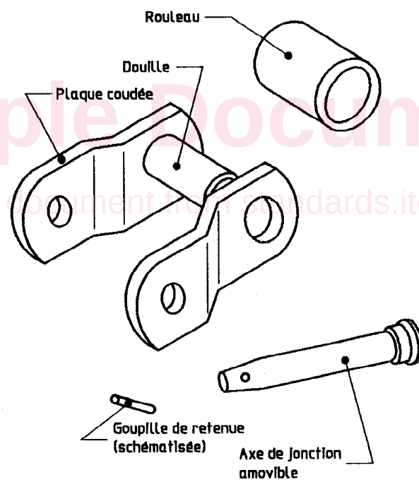
Figure 2 — Éléments d'un maillon coulé
