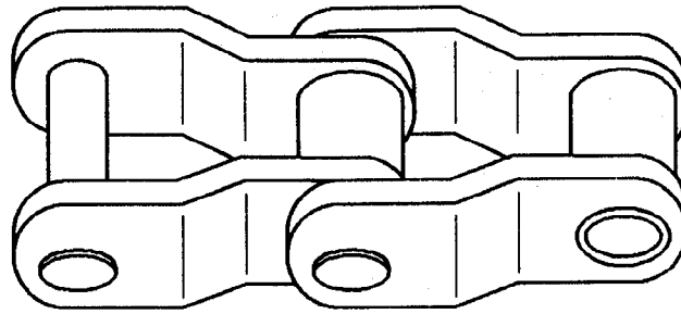
Figure 1 — Chaîne à maillons coulés assemblée
