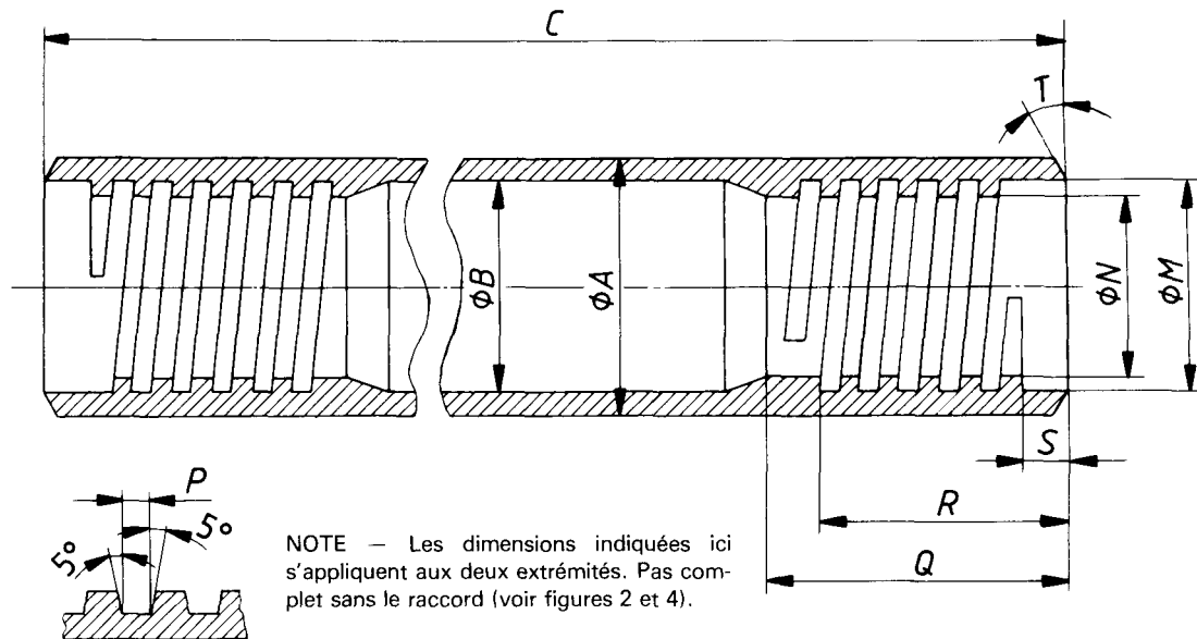
Figure 3 — Tige de forage, modèle W — Tube de la tige de forage (voir tableau 7)
