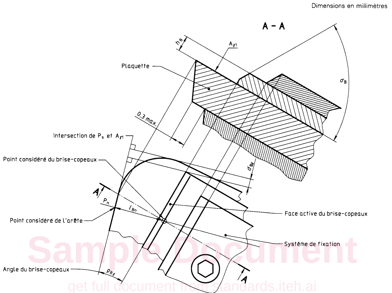
Figure 5 — Dépassement de la plaquette et brise-copeaux
