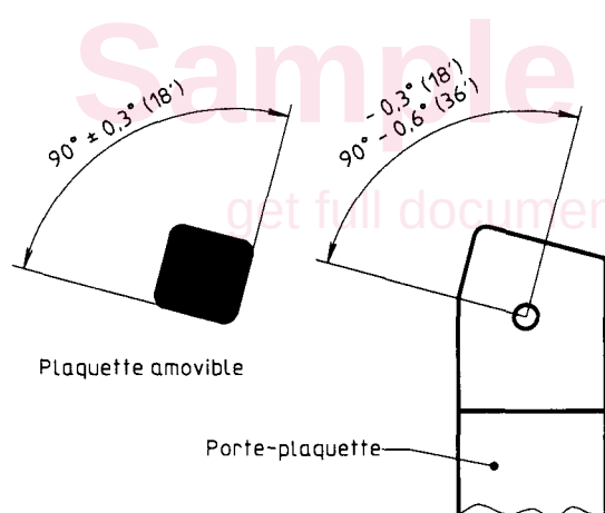
Figure 4 — Tolérances sur l'angle de la plaquette et de son logement
