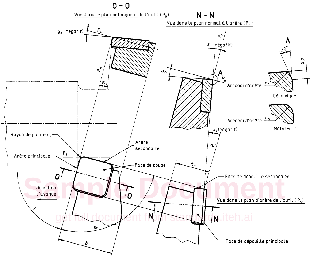
Figure 1 — Illustration des angles de l'outil
