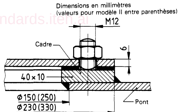
Figure 2 — Type B (trou de main sans surbau)
