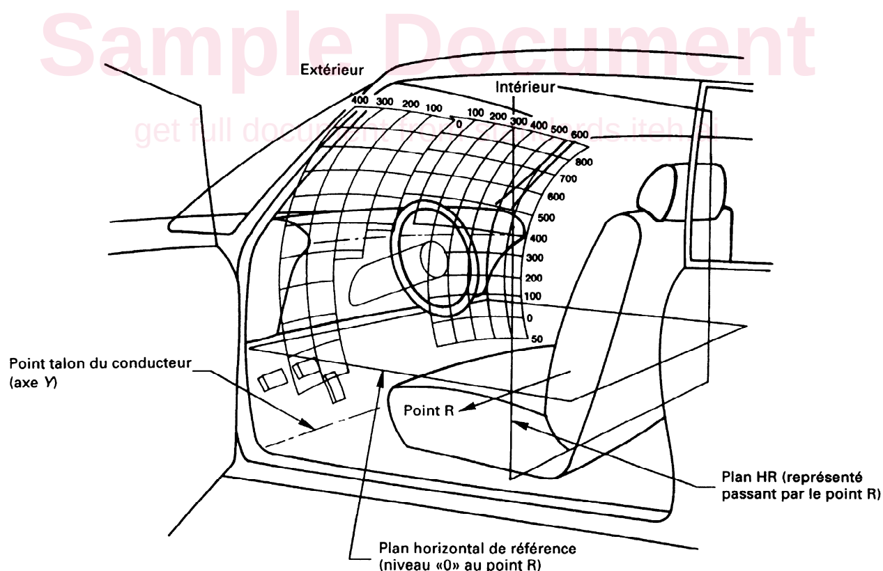
Figure 3 — Enveloppe de portée des mains dans le véhicule
