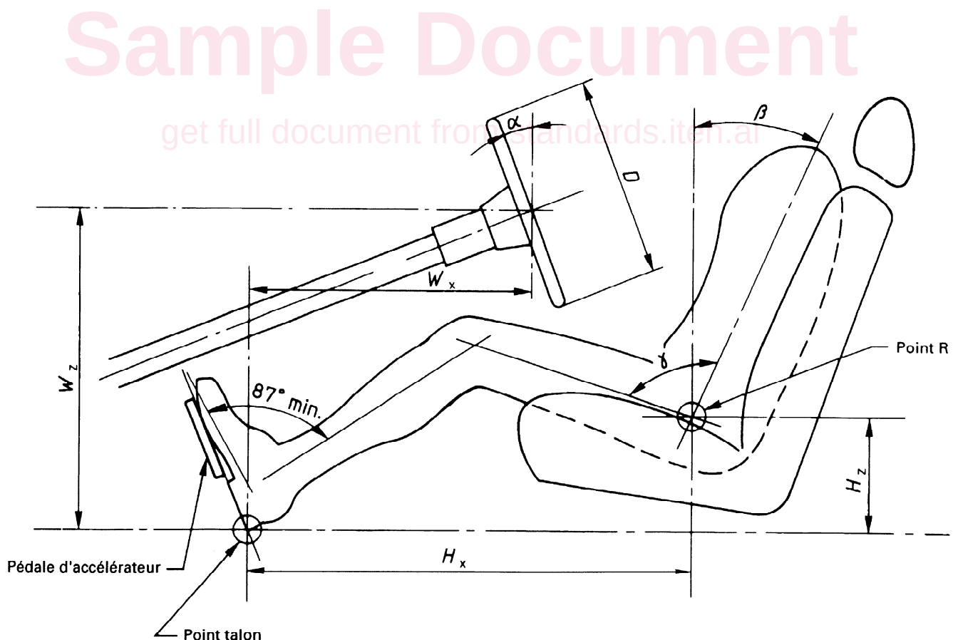
Figure 2 — Dimensions du poste de conduite
