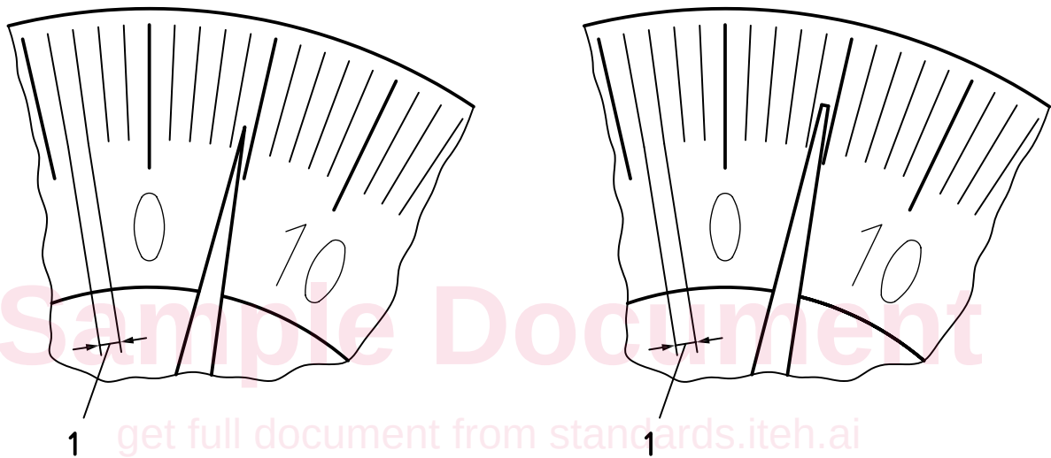
b) Échelle ou cadran où la largeur de la pointe de l'aiguille est inférieure ou égale à 1/5 de la largeur de l'incrément c) Échelle ou cadran où la largeur de la pointe de l'aiguille est supérieure à 1/5 mais inférieure ou égale à 1/2 de la largeur de l'incrément
