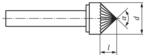
Figure 1 — Fraises-limes en métaux durs, formes J et K
