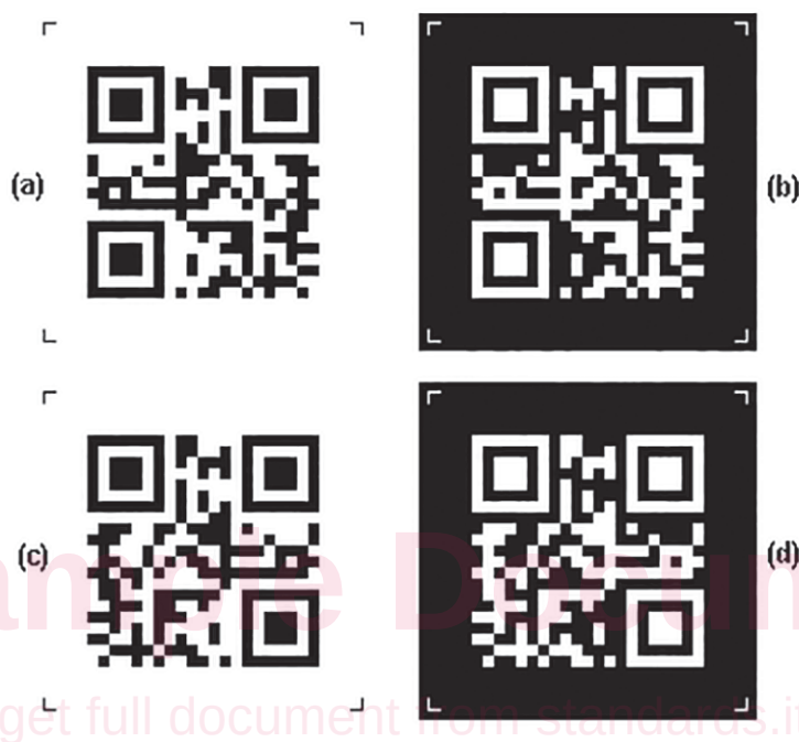
Figure 1 — Exemples de symbole de QR Code codant le texte «symbole de QR Code» – (a) disposition en orientation normale et en réflectance normale; (b) orientation normale et réflectance inversée; (c) orientation en miroir et réflectance normale; (d) orientation en miroir et réflectance inversée
