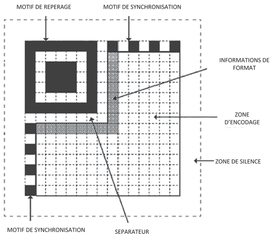
Figure 4 — Structure d'un symbole de Micro QR Code de version M3
