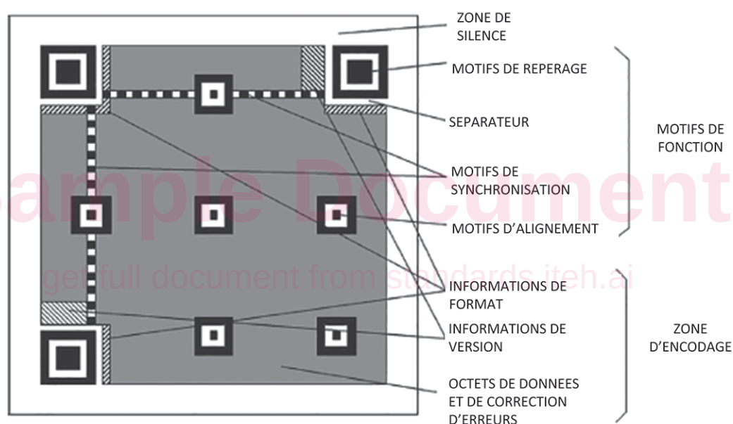
Figure 3 — Structure d'un symbole de QR Code
