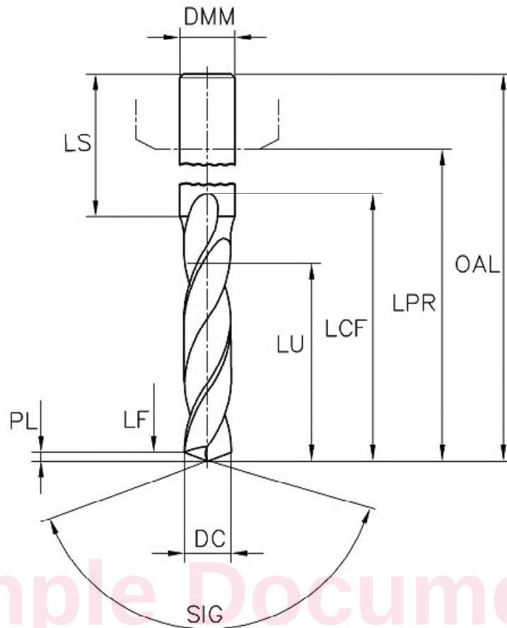
Figure 6 — Foret monobloc — Détermination des propriétés
