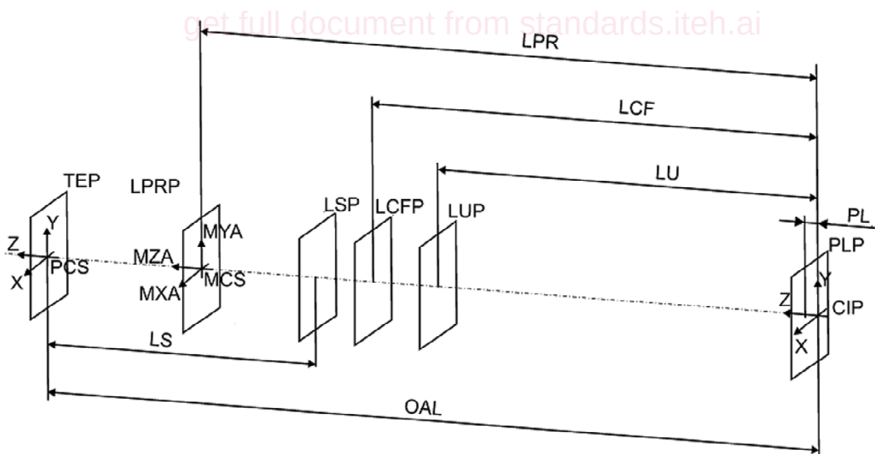
Figure 4 — Plans pour la conception
