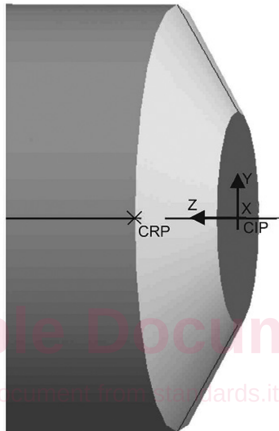
Figure 5 — Position du point de coupe de référence CRP
